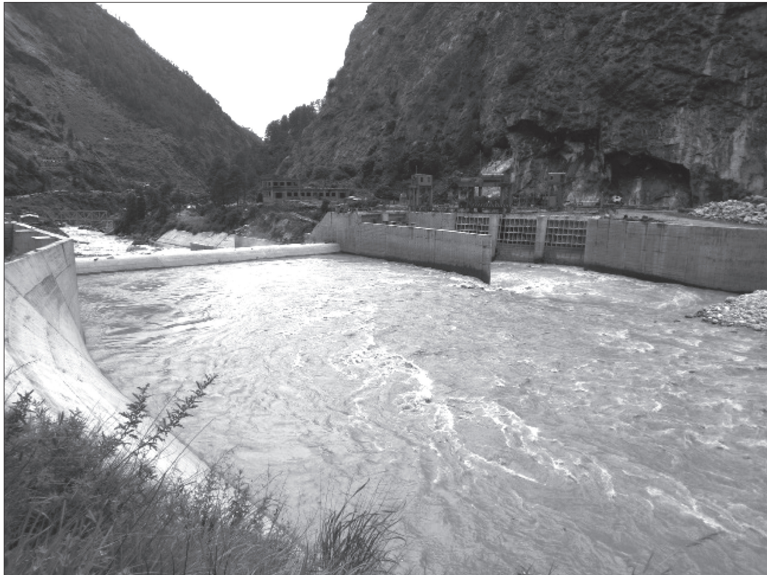
१११ मेगावाट क्षमताको निर्माणाधीन रसुवागढी हाइड्रोपावरले विद्युत् गुहमा पानी लैजान भोटेकोसीमा बाँधेको बाँध । यो बाँधबाट प्रतिसेकेन्ड ८० घनमिटर पानी विद्युत् गुहमा लैजाने आयोजनाको तयारी छ।
